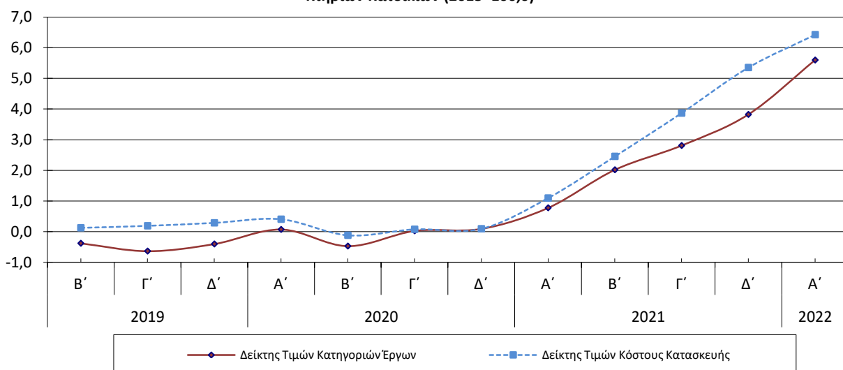
Εξέλιξη ετησίων μεταβολών (%) Δεικτών Τιμών Κατηγοριών Έργων και Κόστους Κατασκευής Νέων Κτηρίων Κατοικιών (2015=100,0)
